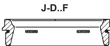
J-D..F kombinierte Docht-/Filzschmierung combined wick/felt lubrication
